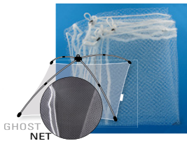
4467 006 Monofil/Ghost-Senknetz 1x1 m / ca. 6 mm Maschenweite Netz: 100 % Nylon.
